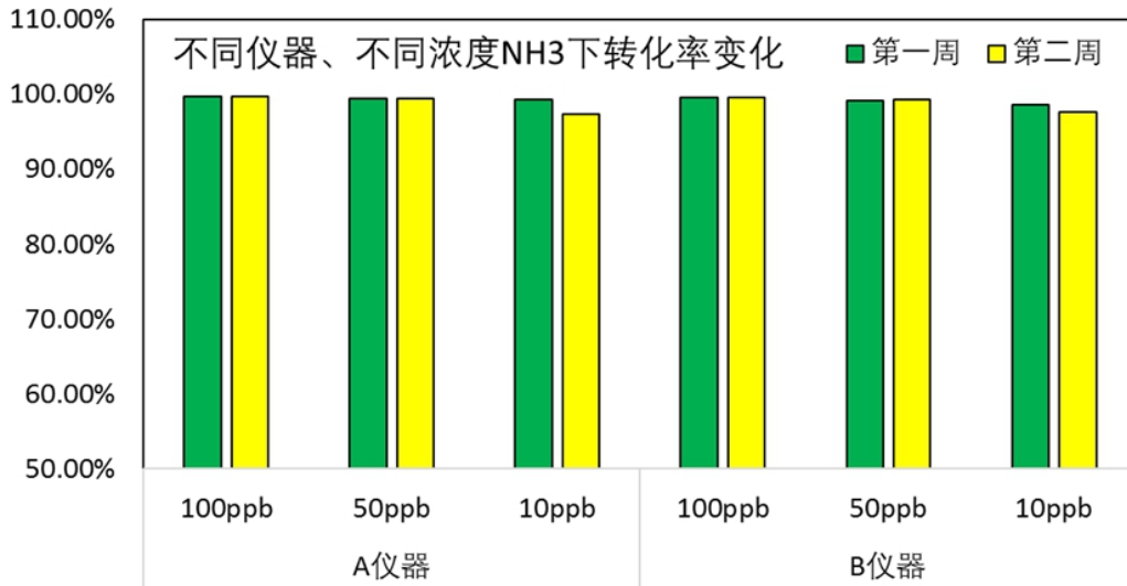
图12 化学发光法氨监测系统转换效率
